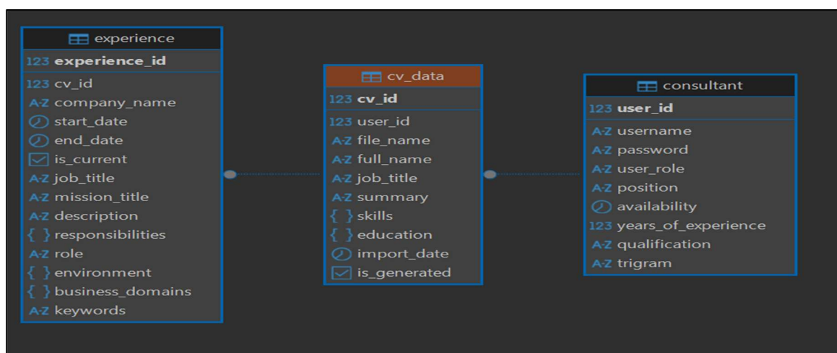
Figure 6. Relation base de données
